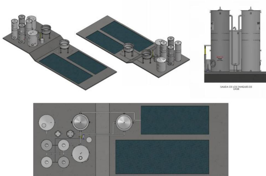
PLANTA DE LIXIVIADOS, CELDA DE CONTINGENCIA DISTRITO BUENAVENTURA (VALLE DEL CAUCA).
